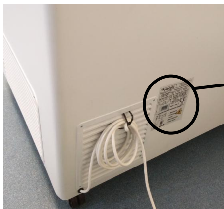
Fig. 13 - Emplacement de la plaque signalétique
