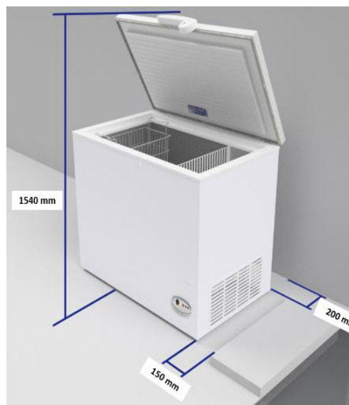
Fig. 4 - Distancias mínimas de instalación
